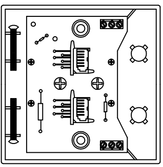
PCB板 銅箔: 2oz/1oz
