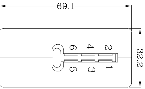
FR PLUG(P1)
